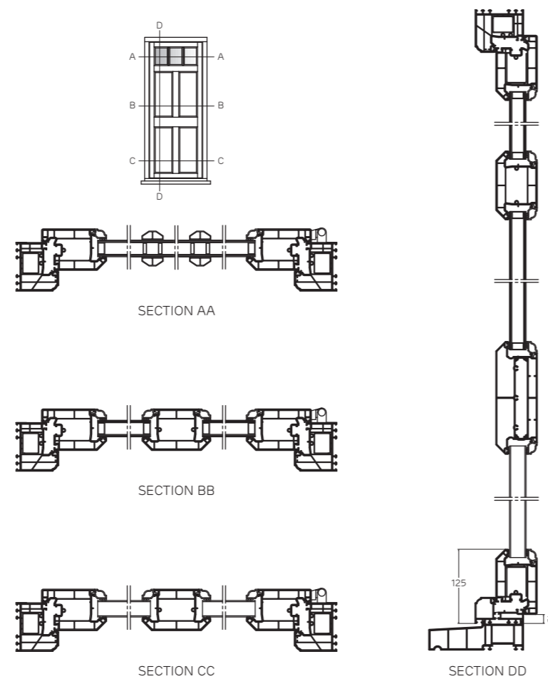
The English Door Ballington Door
